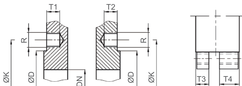
DN 80-200
